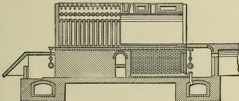
FIG. 92.—Koppers Coke-oven.
